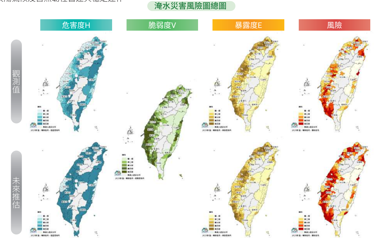
(附圖說明)：篩選高度影響之據點，研究結果顯示淹水為新東陽最需預防之災害。
